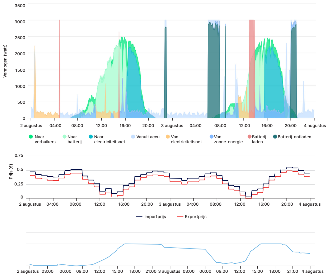
SolarEdge ONE batterijoptimalisatie in een residentiële site in Nederland, met een dynamisch energiecontract.
